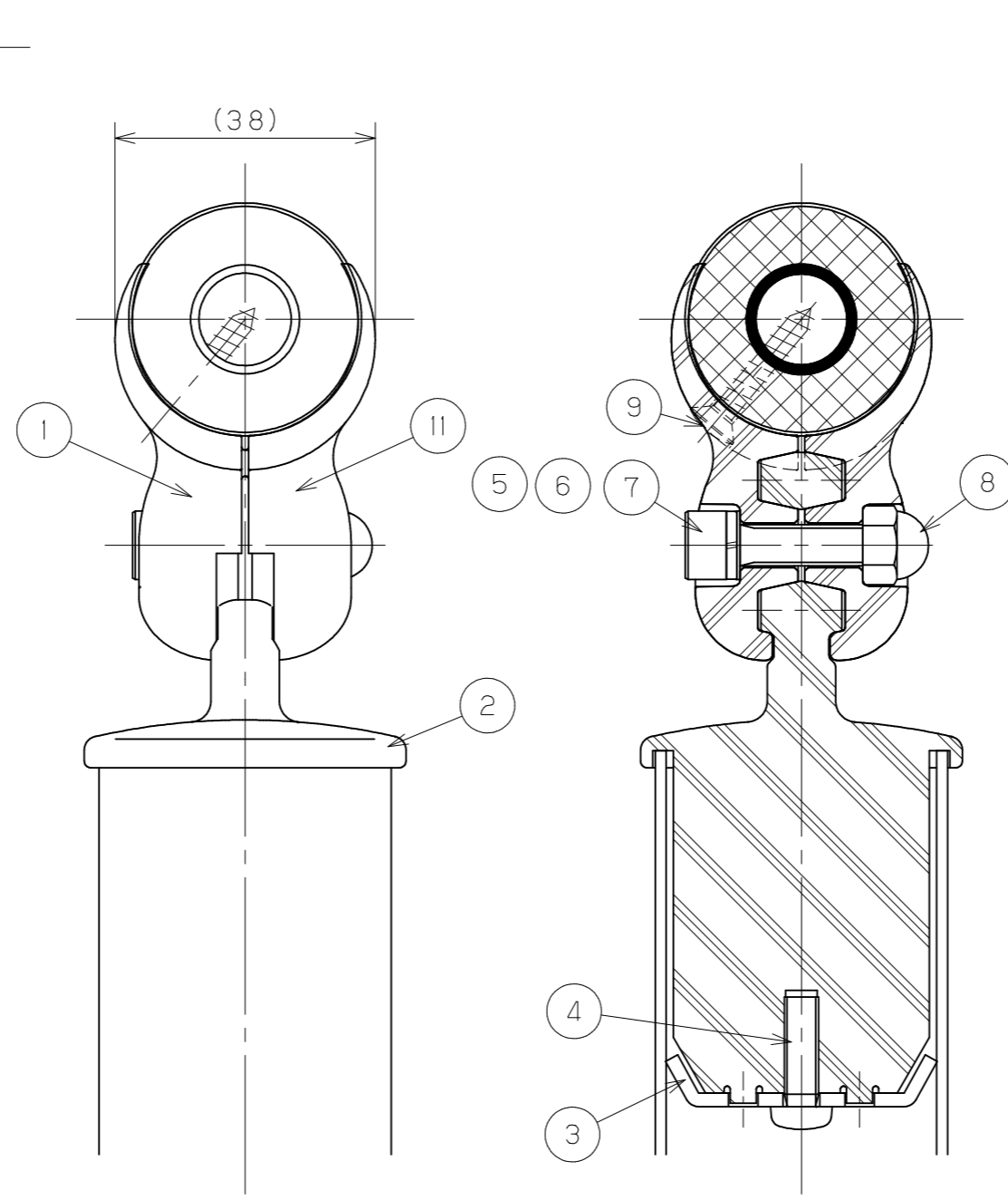
A-A断面図
